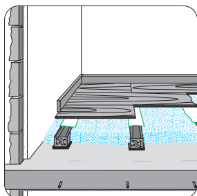
Aufbau Nr.: Bo-20 x
