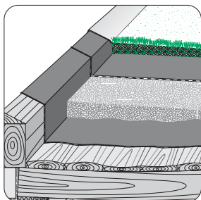
Aufbau Nr.: Da-81
