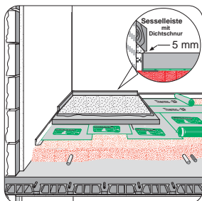
Aufbau Nr.: Bo-4
