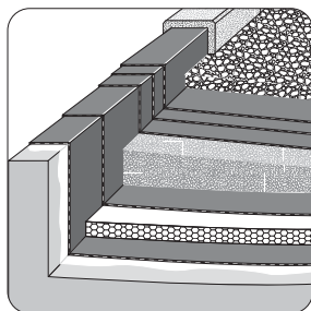
Aufbau Nr.: Da-40 sa
