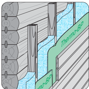
Aufbau Nr.: Wa-14
