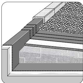
Aufbau Nr.: Da-41
