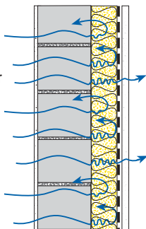
1c dichter Vollwärmeschutz
