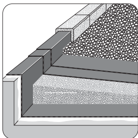
Aufbau Nr.: Da-40
