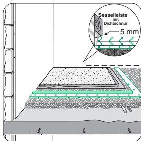
Aufbau Nr.: Bo-10
