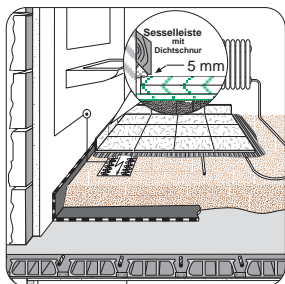
Aufbau Nr.: Bo-10 n
