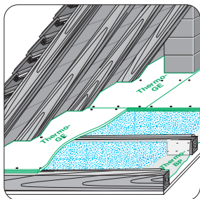
Aufbau Nr.: De-41
