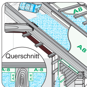
Aufbau Nr.: Da-1 sa
