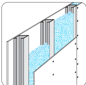
Aufbau Nr.: Wa-61
