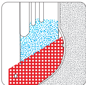
Aufbau Nr.: In-30 st
