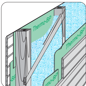
Aufbau Nr.: Wa-51
