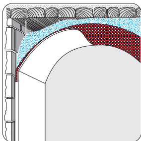
Aufbau Nr.: De-5
