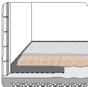
Aufbau Nr.: Bo-32
