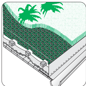
Aufbau Nr.: Da-70
