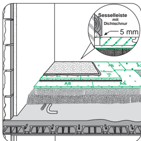
Aufbau Nr.: Bo-13
