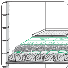
Aufbau Nr.: De-10 mit Bo-11
