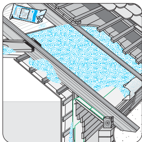
Aufbau Nr.: Da-10, 11
