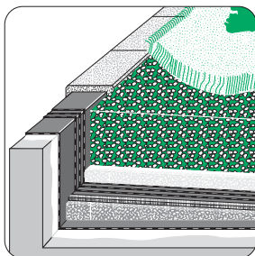
Aufbau Nr.: Da-80
