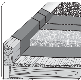
Aufbau Nr.: Da-50
