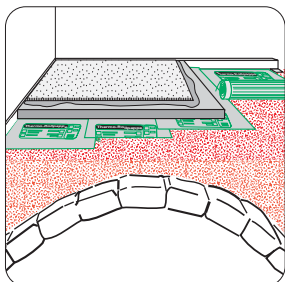
Aufbau Nr.: De-30 mit Bo-1
