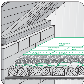
Aufbau Nr.: De-42 bis -45
