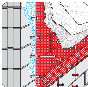
Aufbau Nr.: Wa-1
