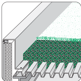
Aufbau Nr.: Da-81 b
