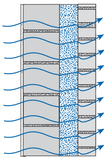
1d offene Kerndämmung
