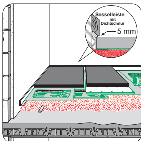
Aufbau Nr.: Bo-3,-3 a8
