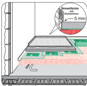
Aufbau Nr.: Bo-1
