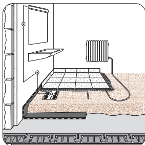
Aufbau Nr.: Bo-31 a
