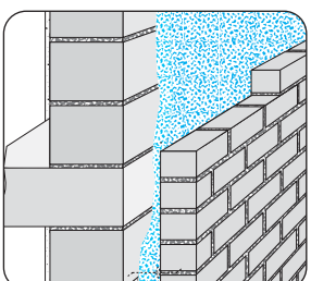
2-schalige Wand Kerndämmung
