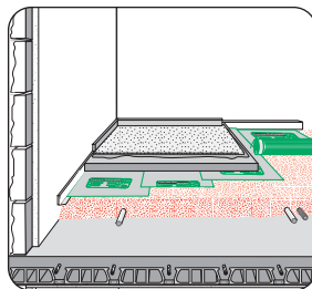
Fließestrich
