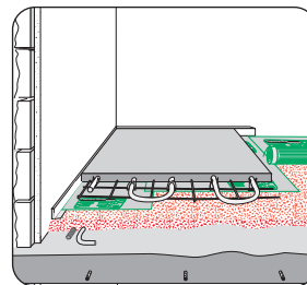
Fußbodenheizung
