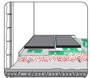
Asphaltestrich
