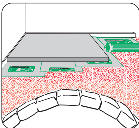
Zementestrich
